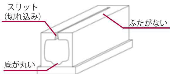
スリット側溝の構造図
