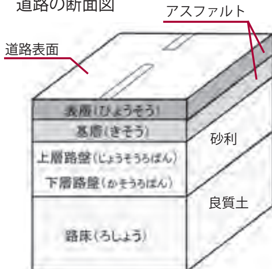
道路の断面図
