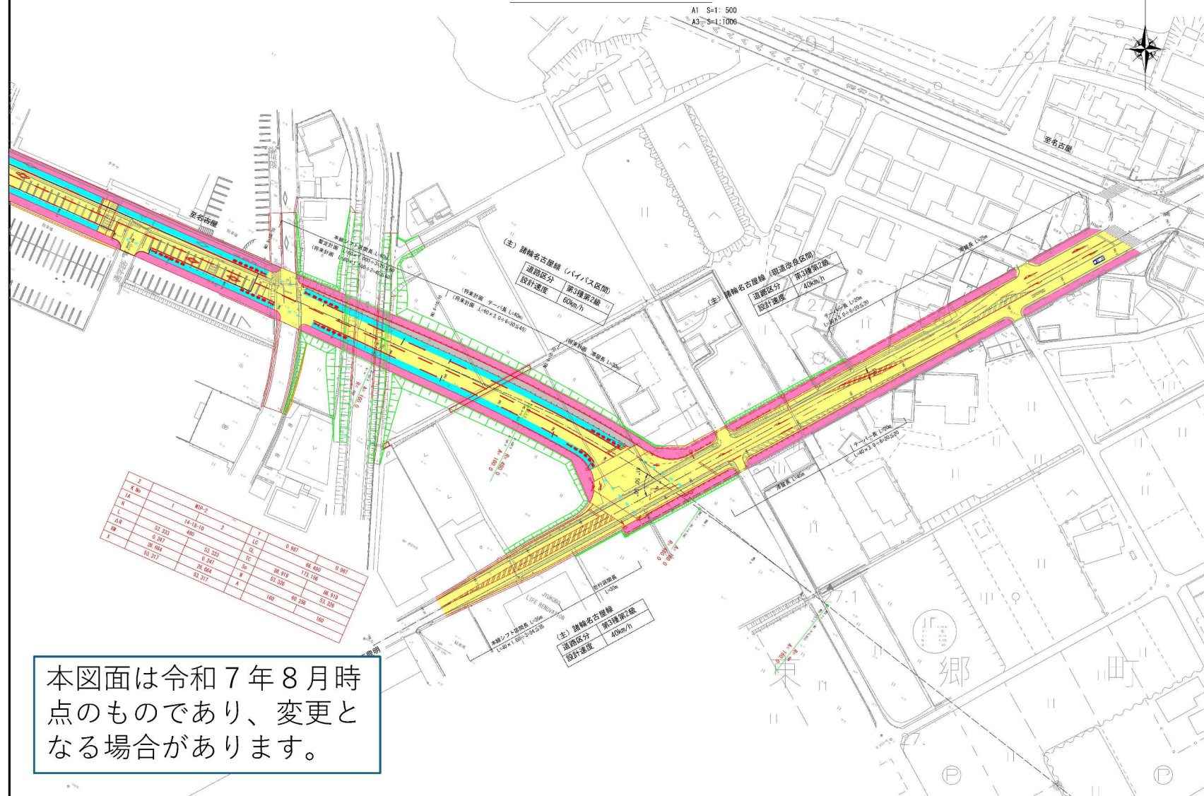
道路整備平面図(2)
